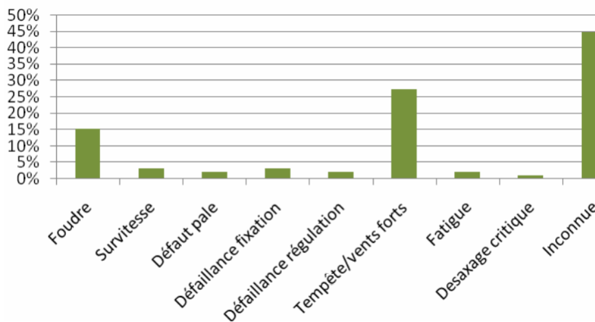
Figure 12 - Répartition des causes premières de rupture de pale, SER-FEE 2012
