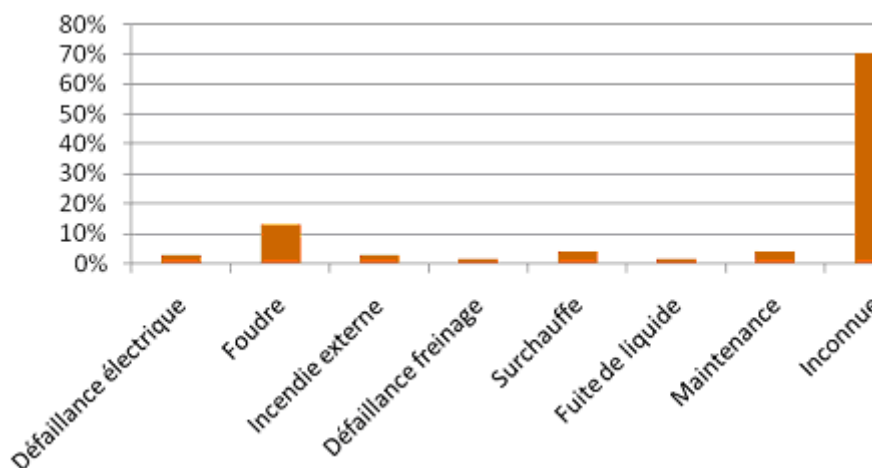
Figure 13 - Répartition des causes premières d'incendie, SER-FEE 2012
