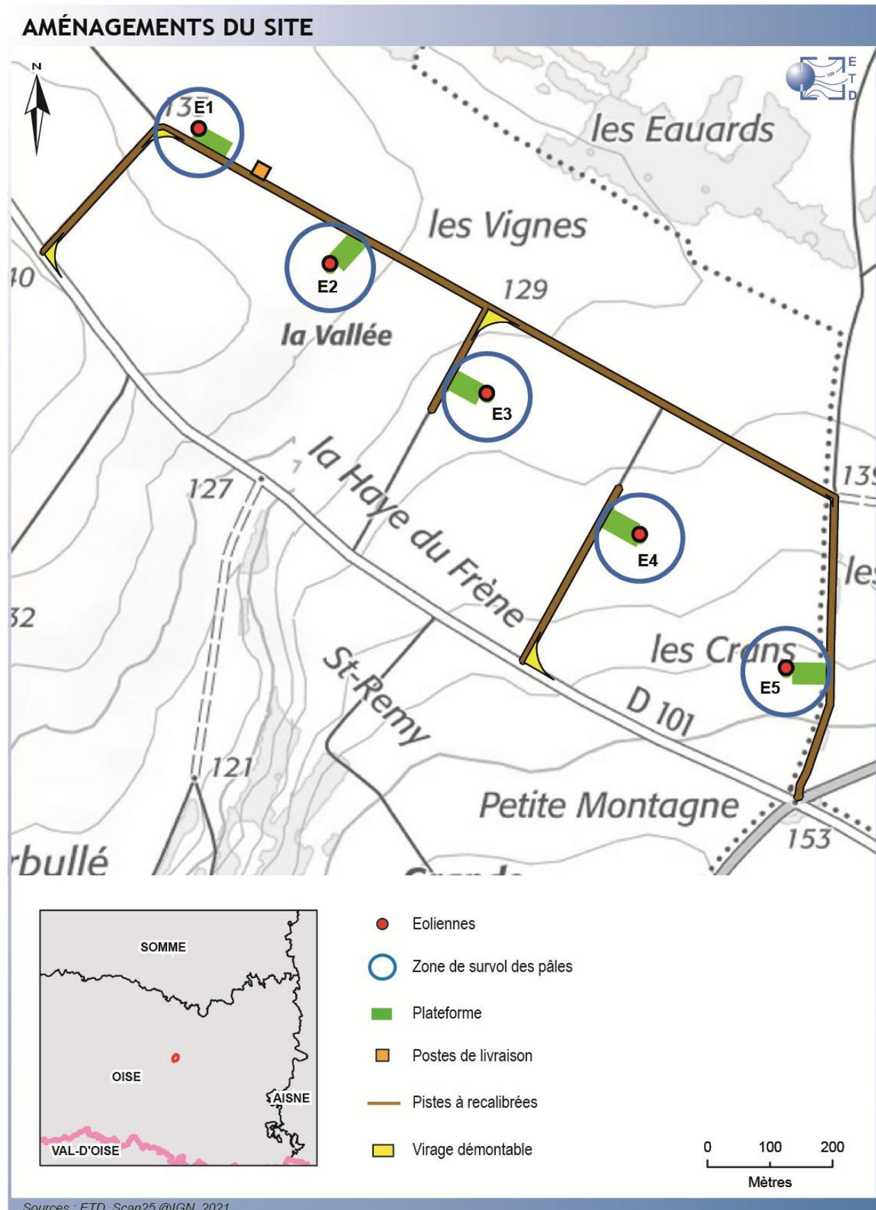
Carte 12 - Plan détaillé de l'installation
